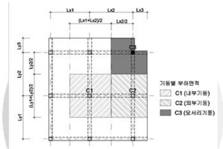
그림 1.4-1 기둥의 부하면적
