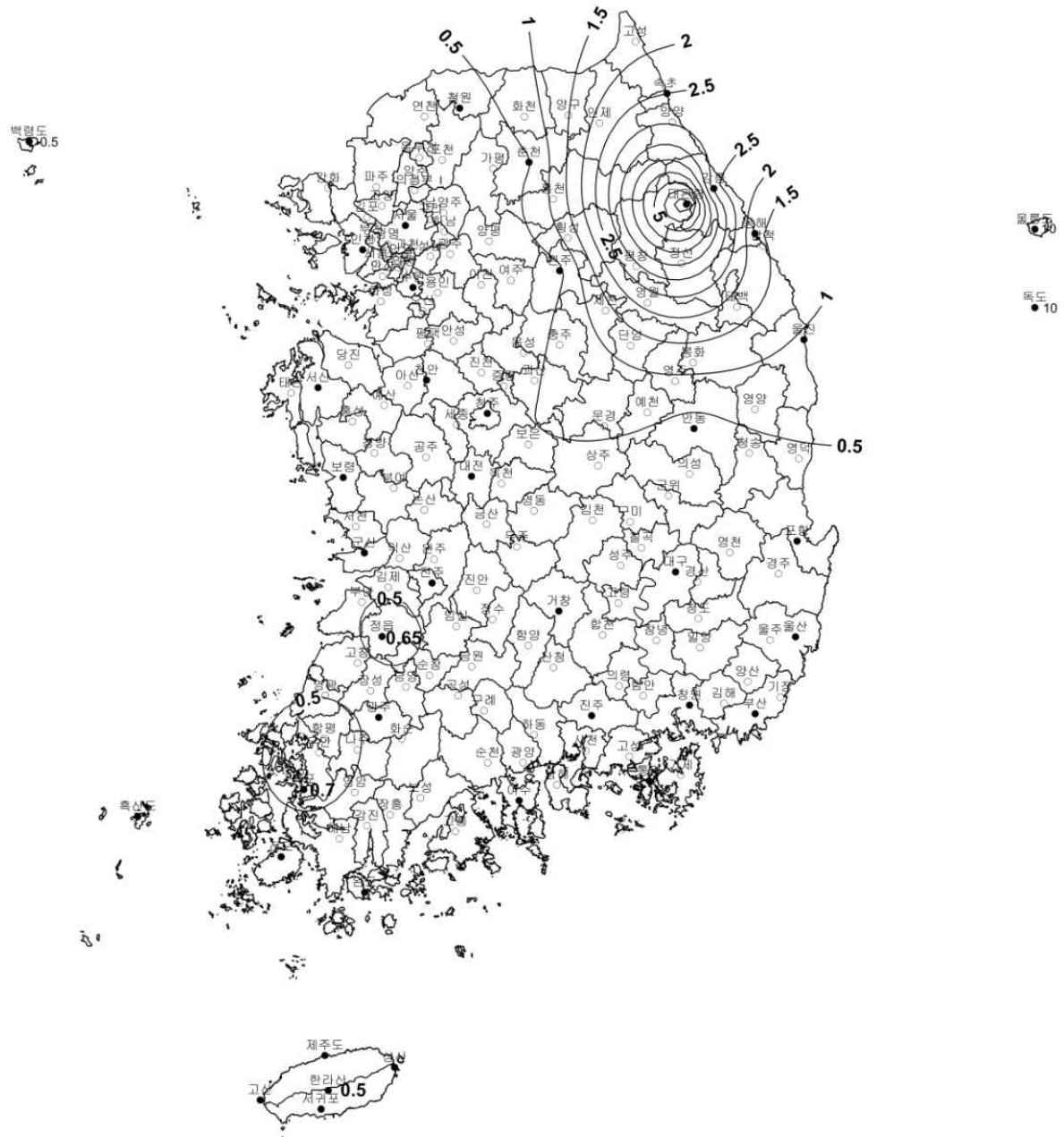
그림 1.2-1 기본지상적설하중 S_g (kN/m 2 )
